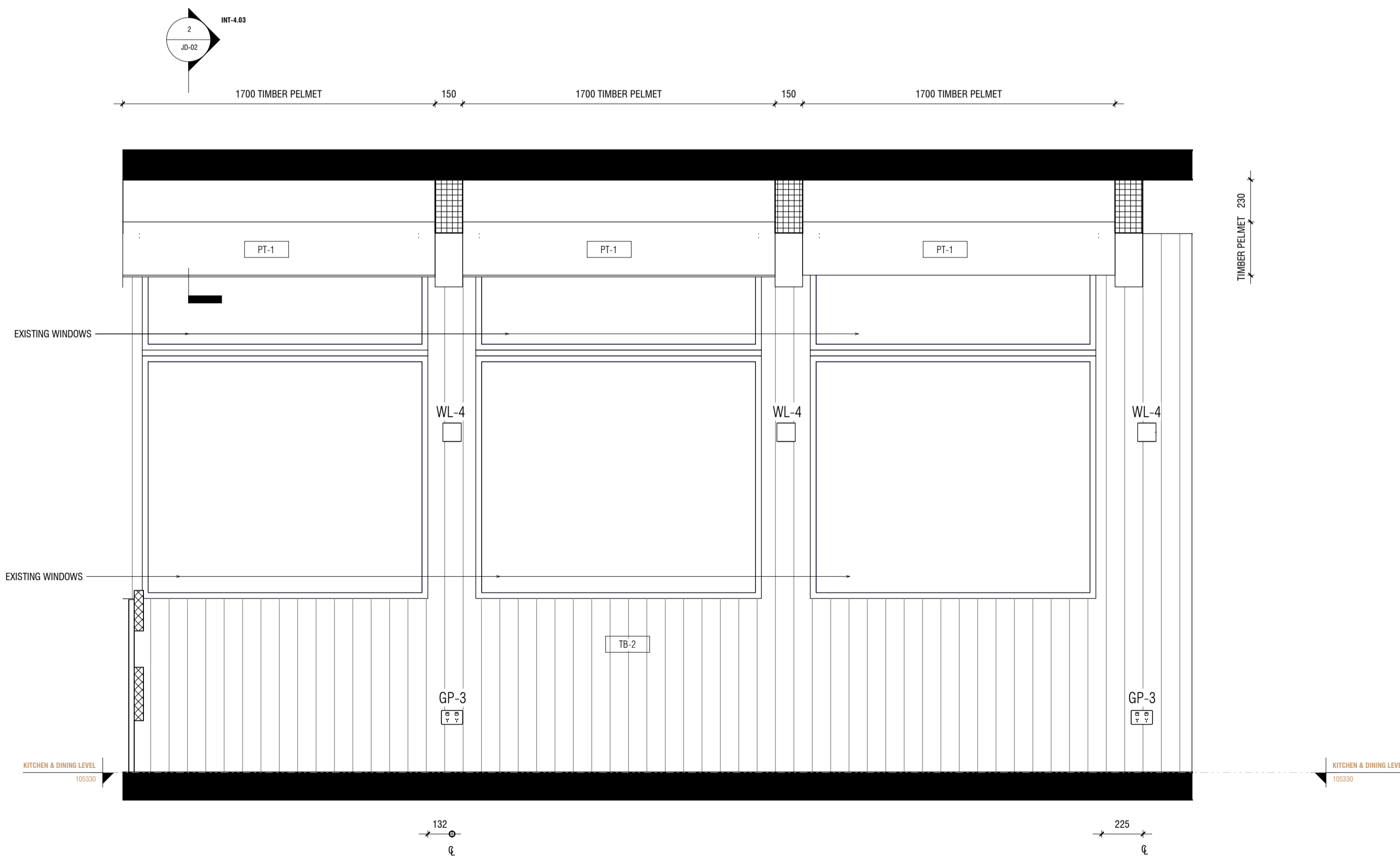
1 INT-4.03 ELEVATION 1 1:20
