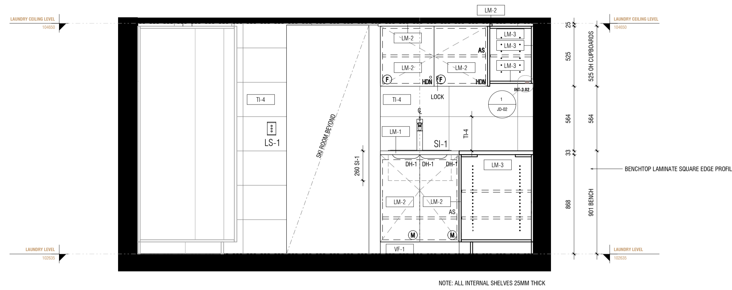
3 INT-6.02 ELEVATION 3 1 : 20
