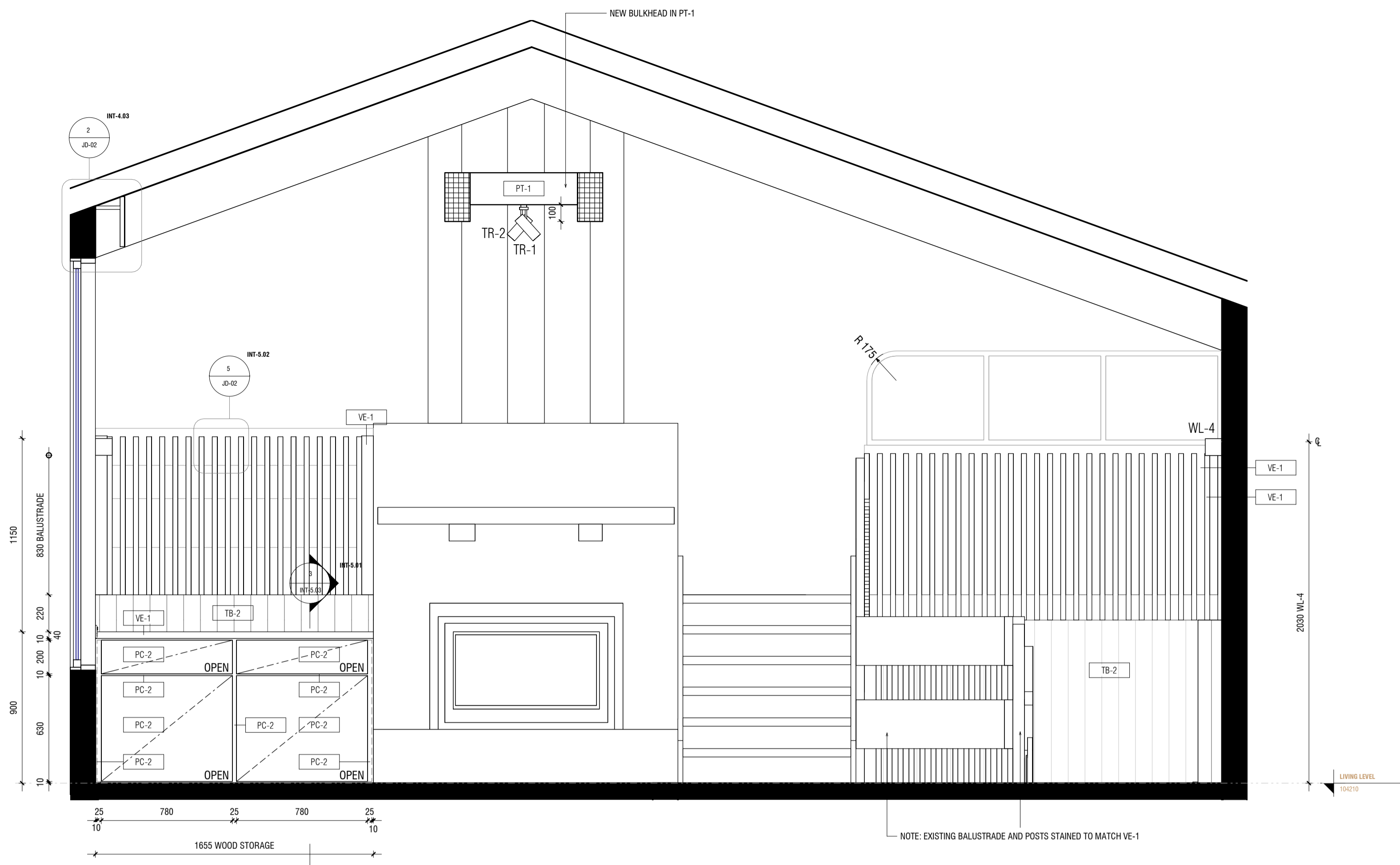
1 INT-5.02 ELEVATION 1 1 : 20
