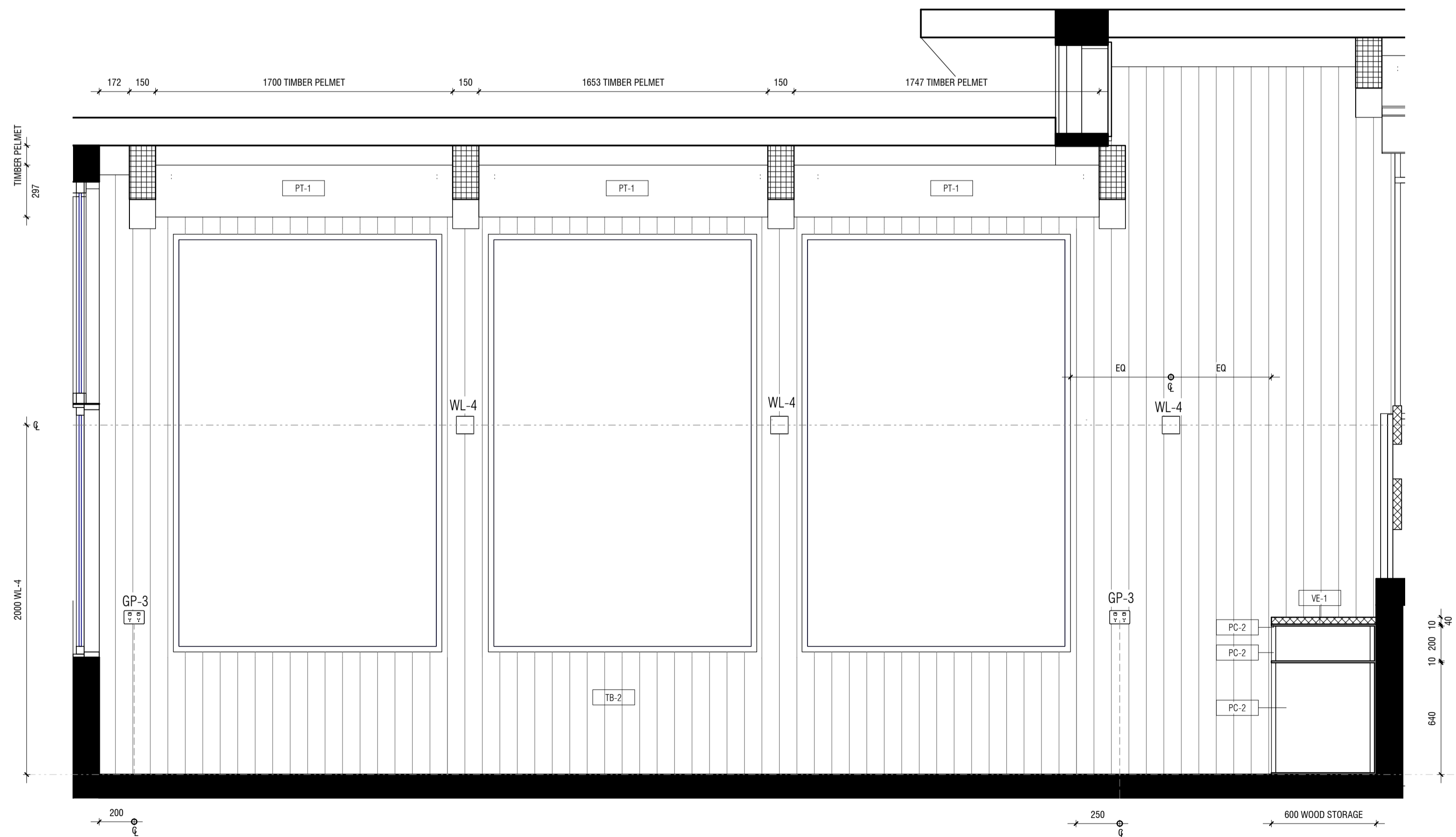
2 INT-5.03 ELEVATION 2 1:20
