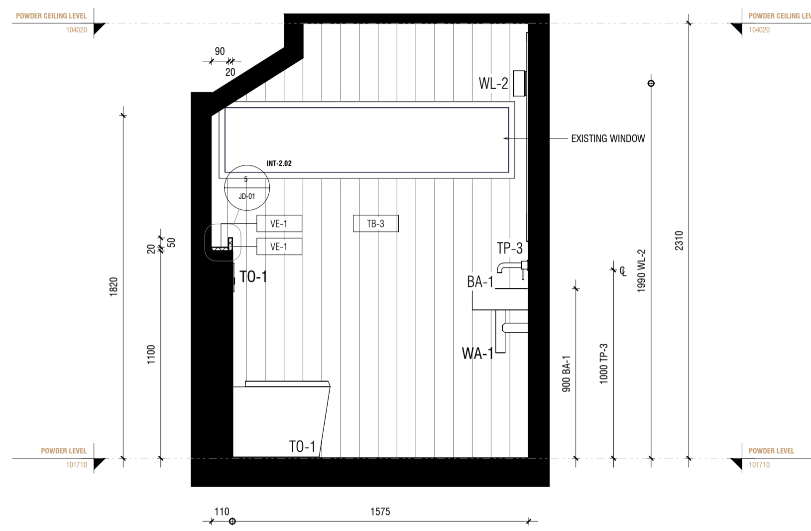
3 INT-7.02 ELEVATION 3 1:20
