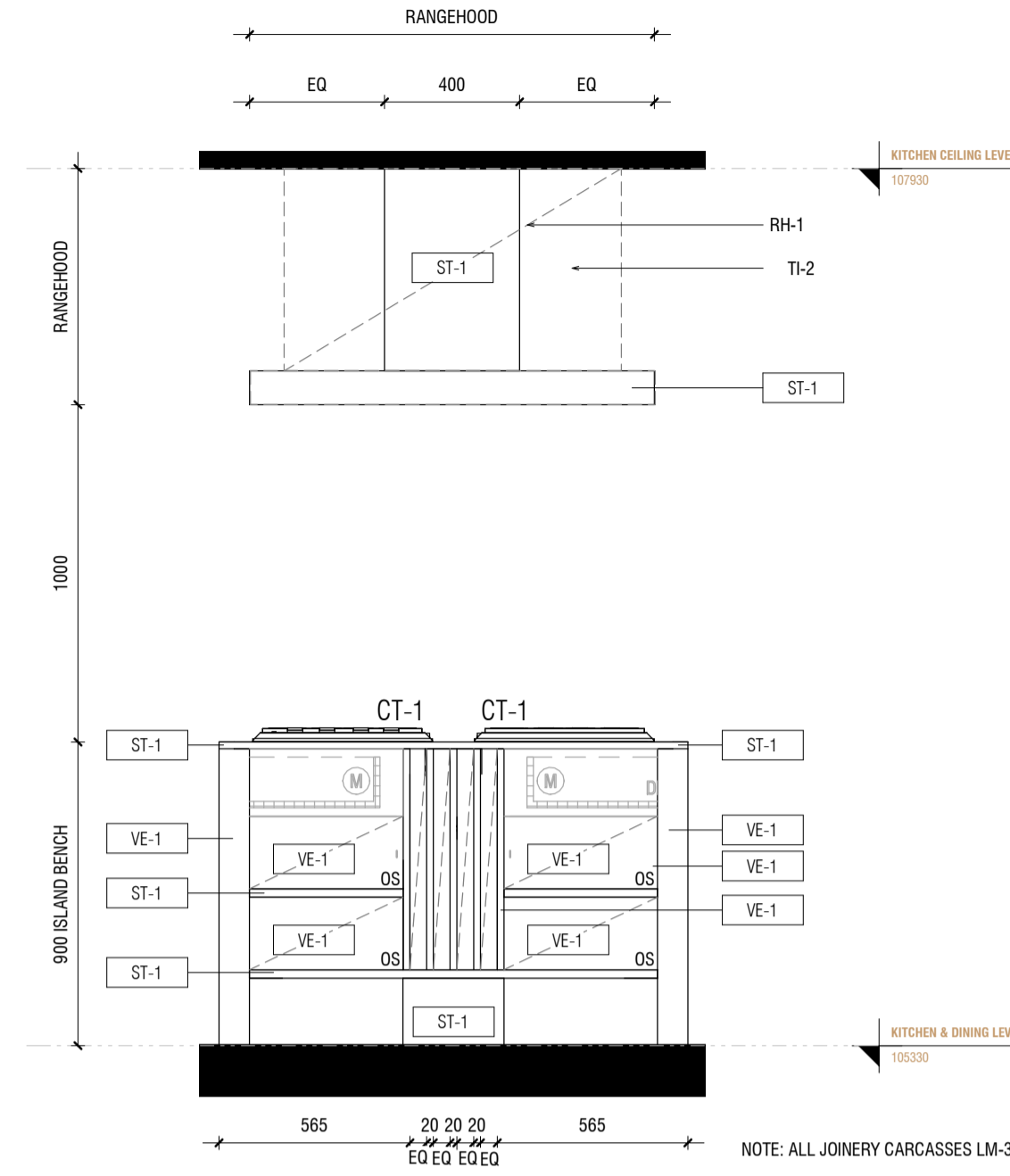
3 INT-3.05 ELEVATION 3 1 : 20
