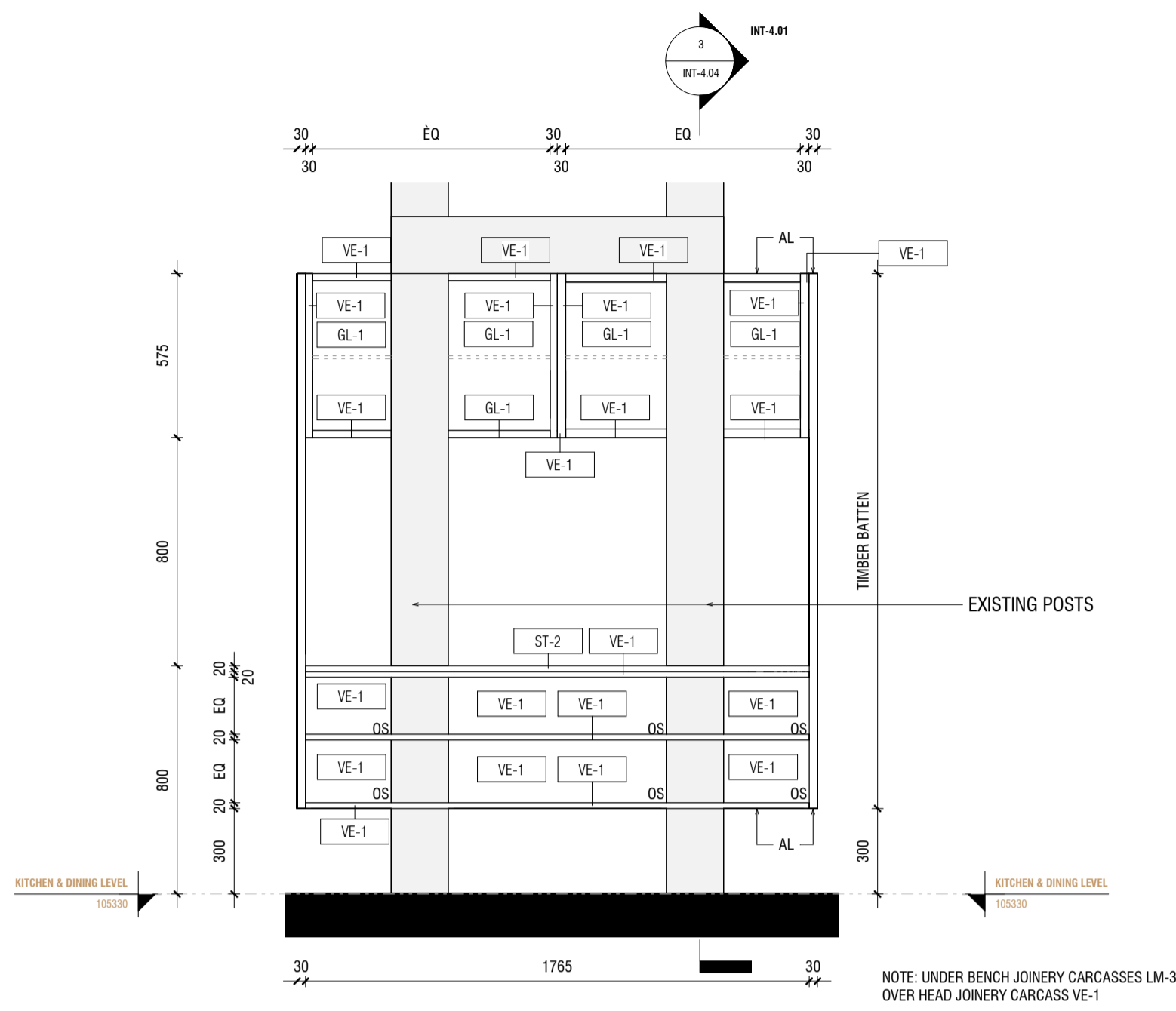
1 INT-4.04 ELEVATION 1 1 : 20
