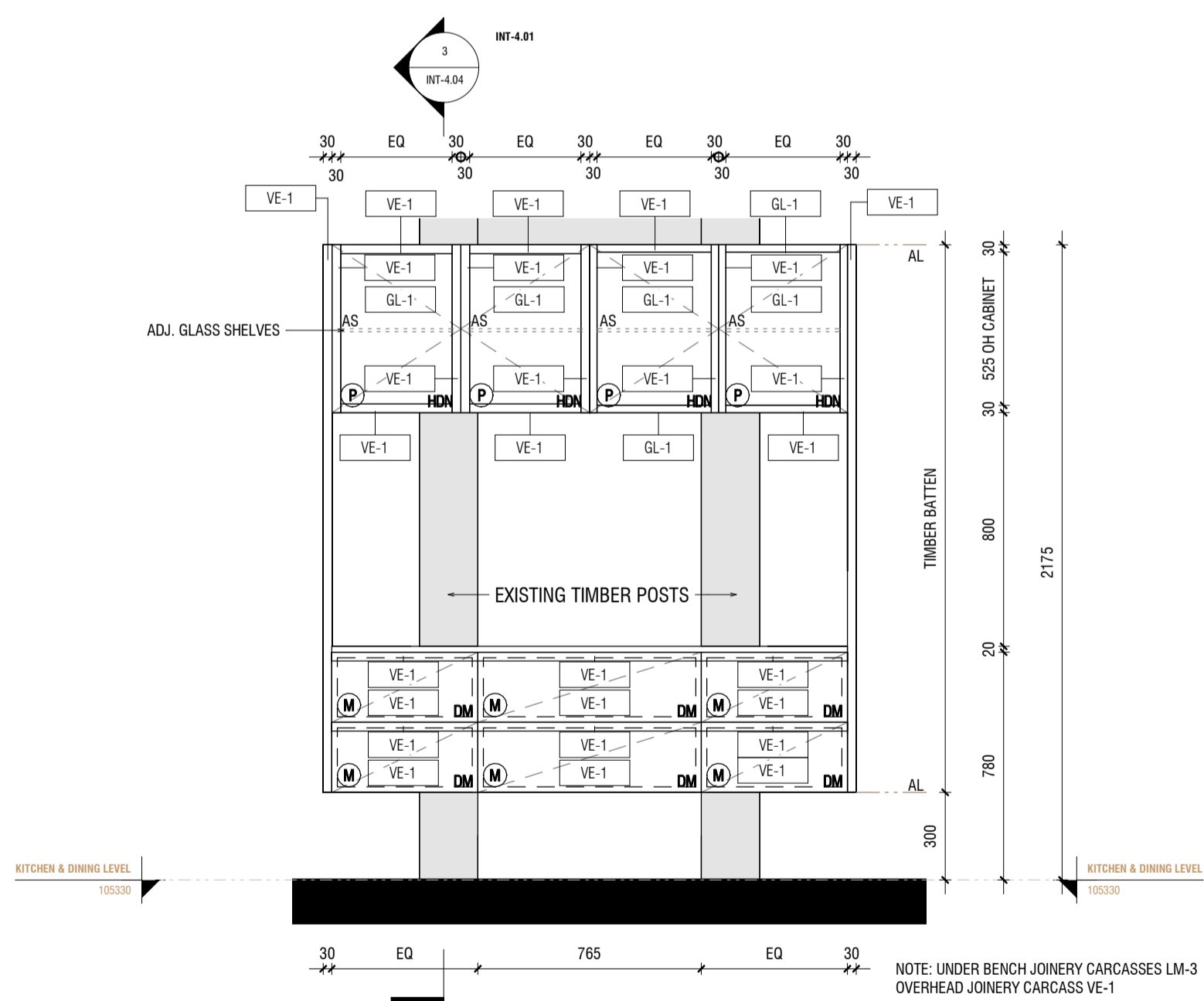
2 INT-4.04 ELEVATION 2 1 : 20
