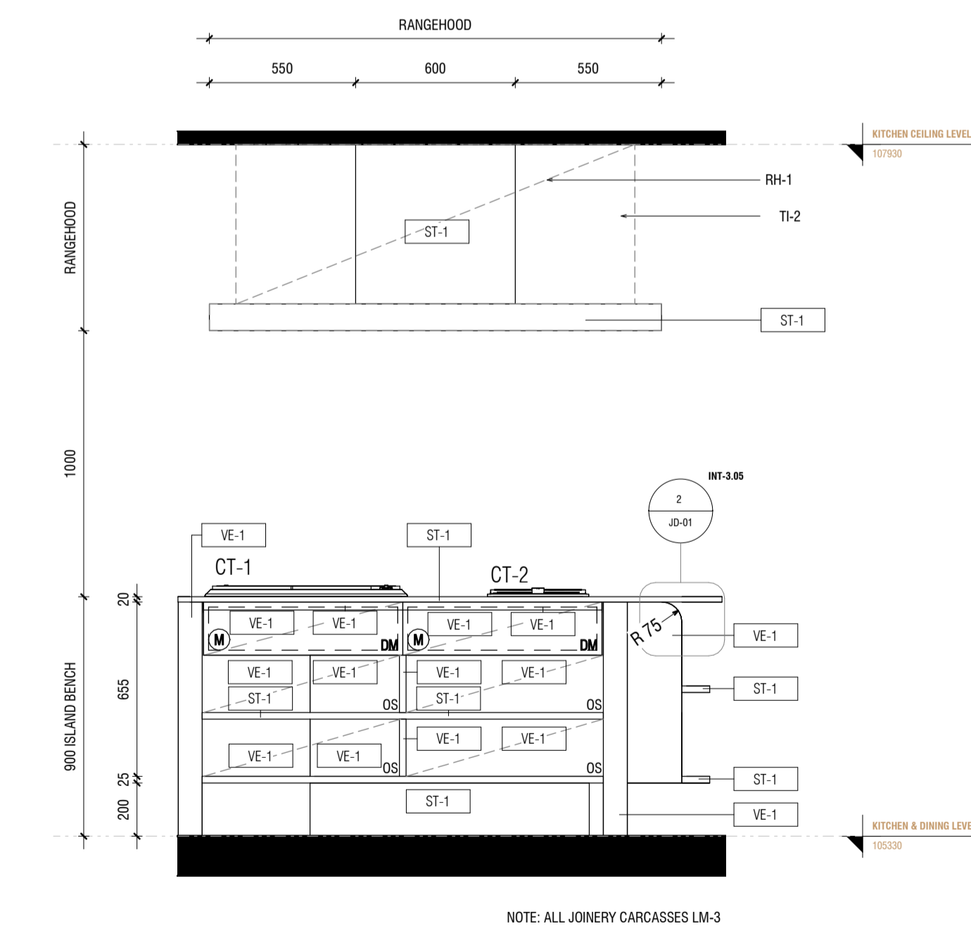
2 INT-3.05 ELEVATION 2 1 : 20
