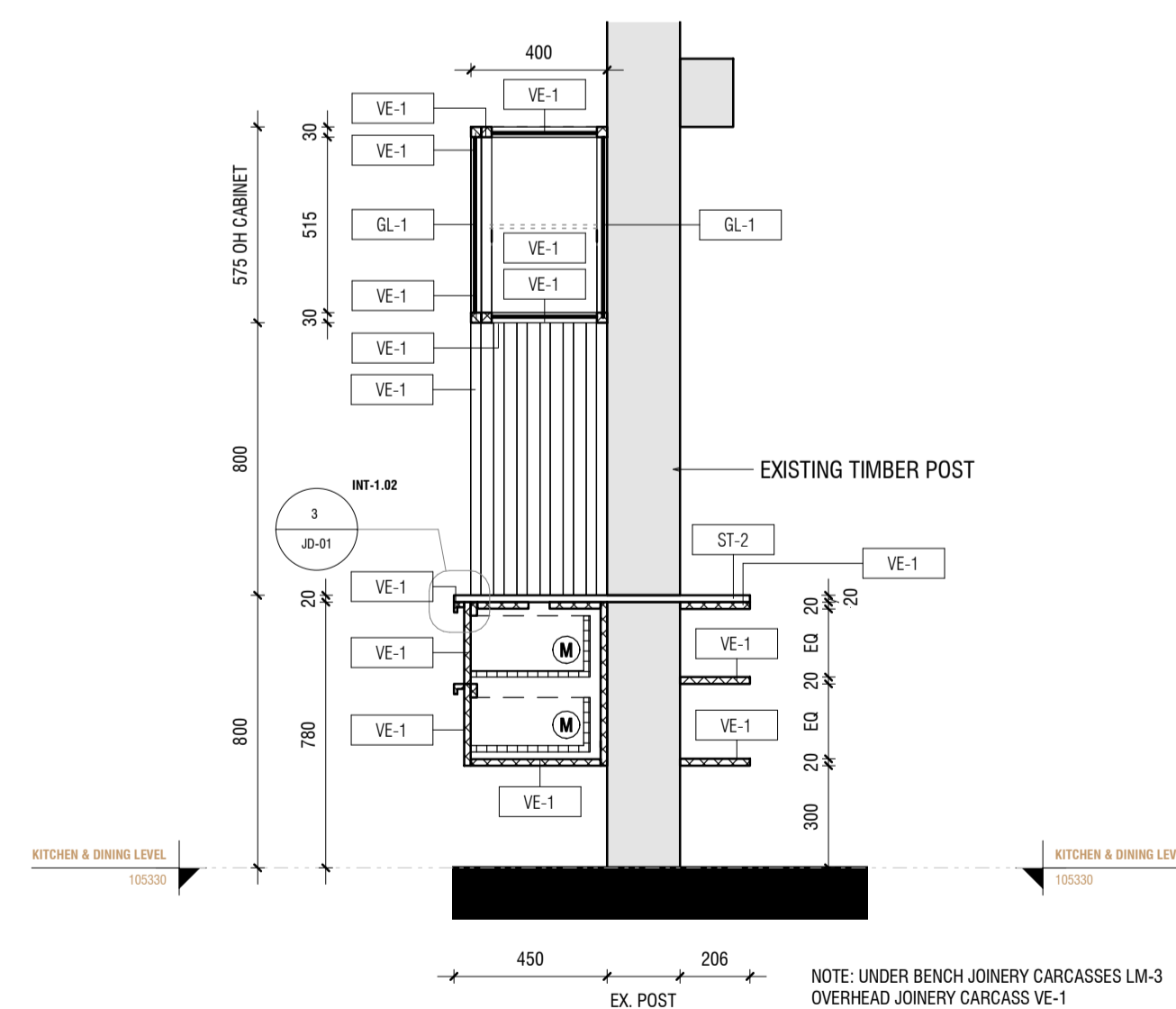
3 INT-4.04 SECTION 1 1 : 20
