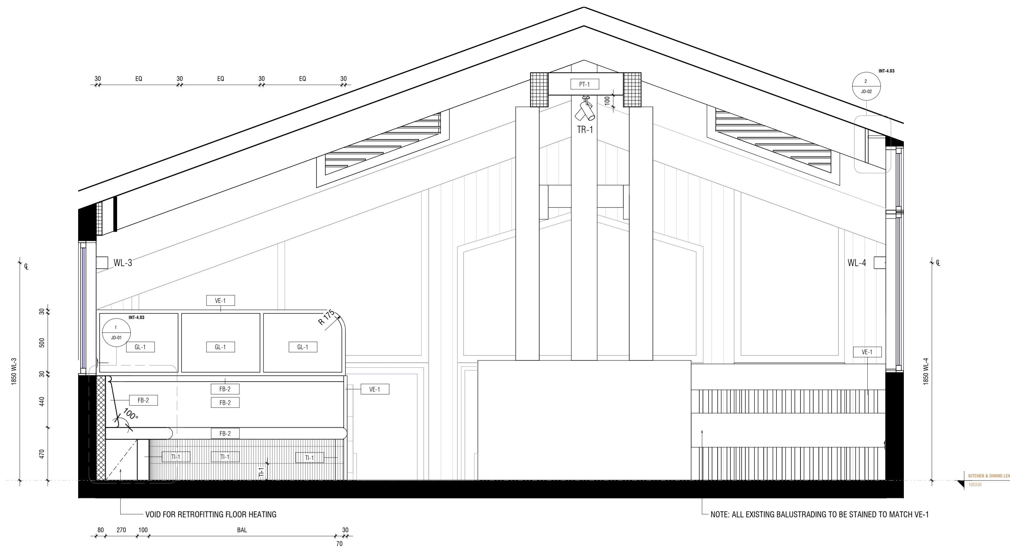
1 INT-4.03 ELEVATION 1 1:20
