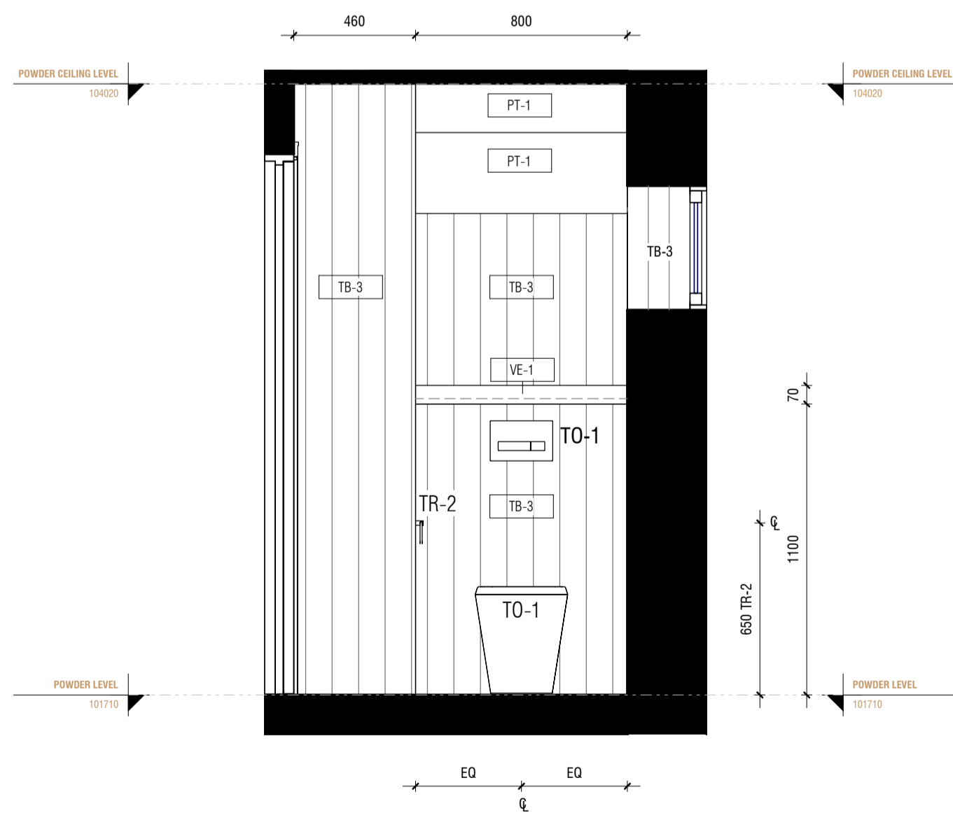
2 INT-7.02 ELEVATION 2 1:20
