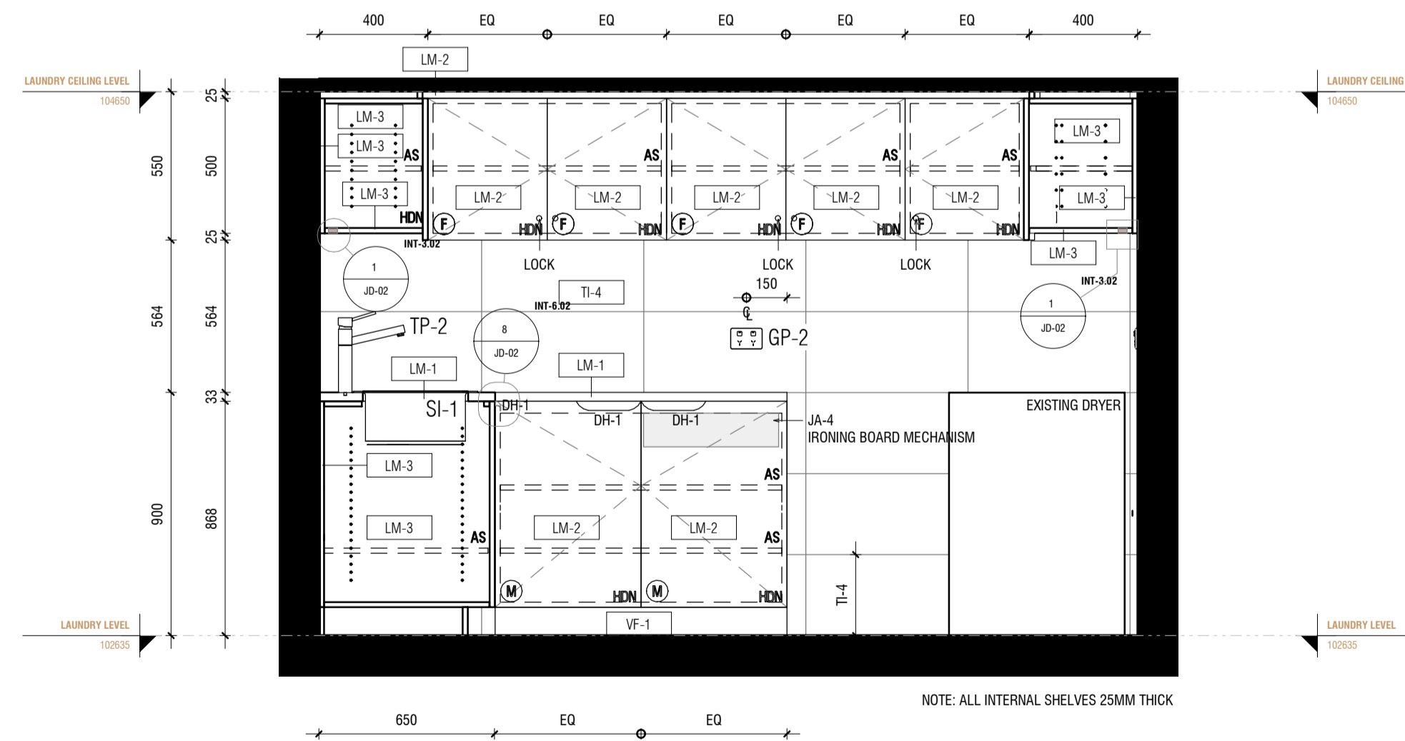
4 INT-6.02 ELEVATION 4 1 : 20
