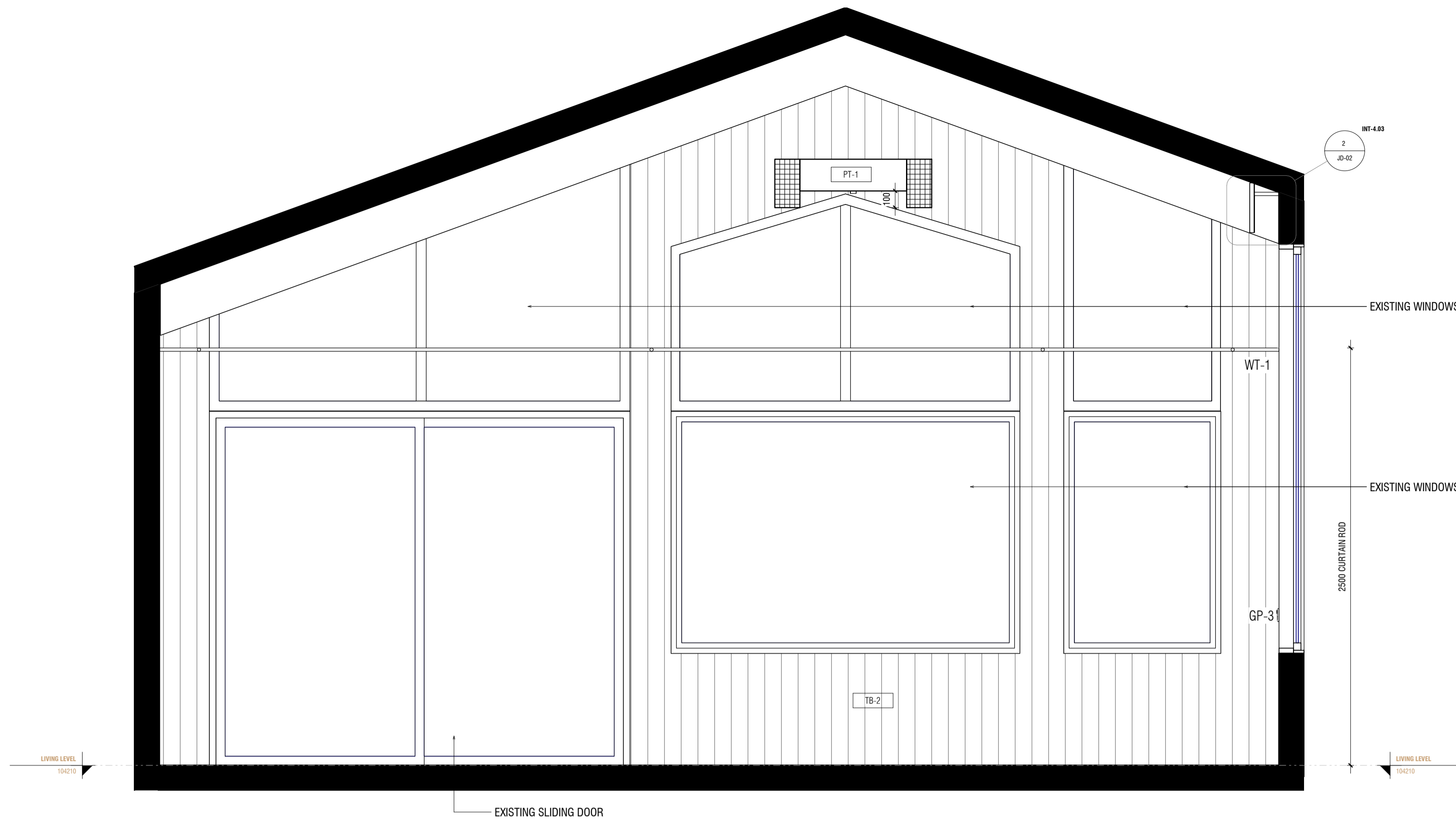
1 INT-5.03 ELEVATION 1 1:20
