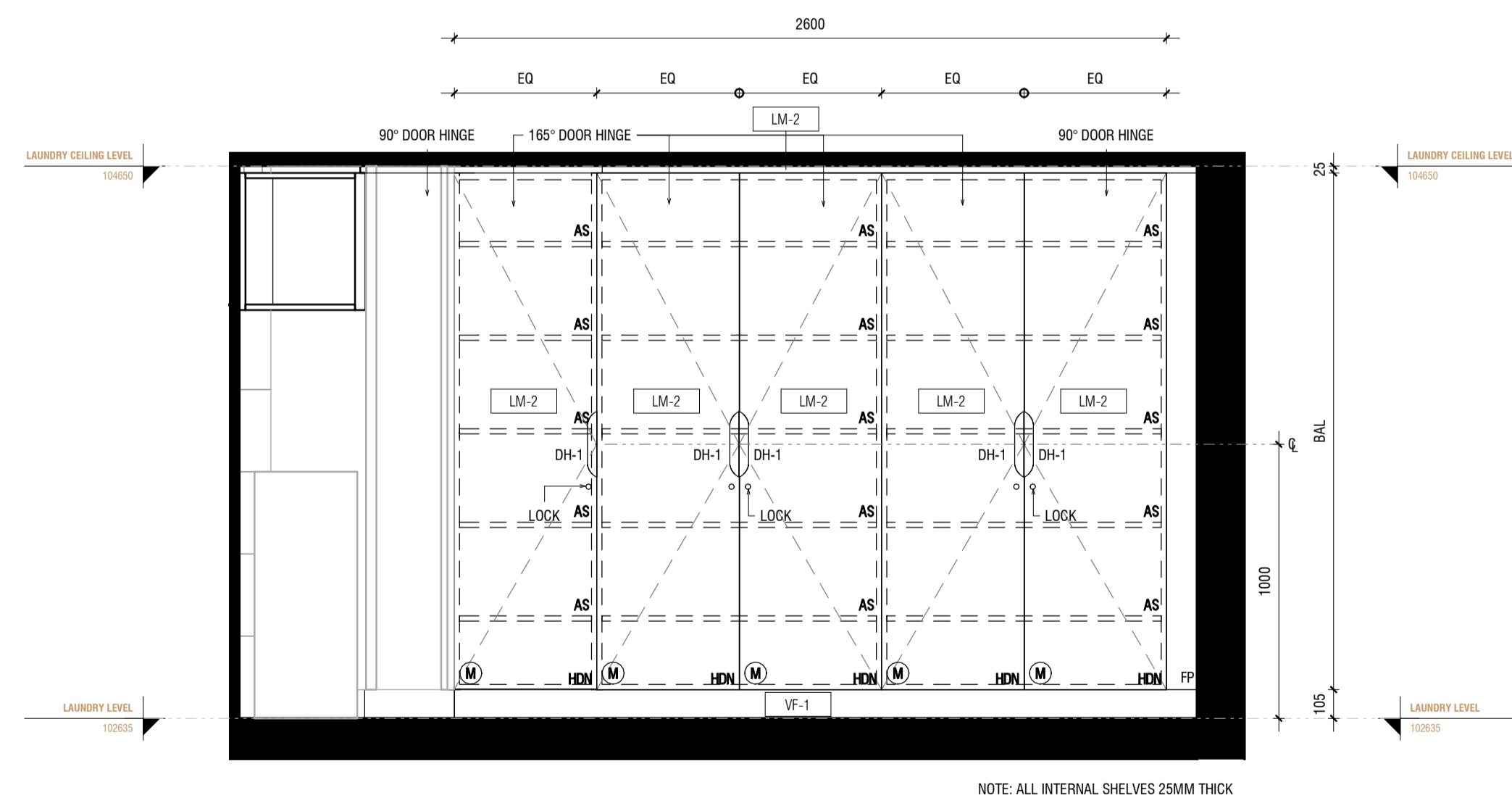
2 INT-6.02 ELEVATION 2 1 : 20
