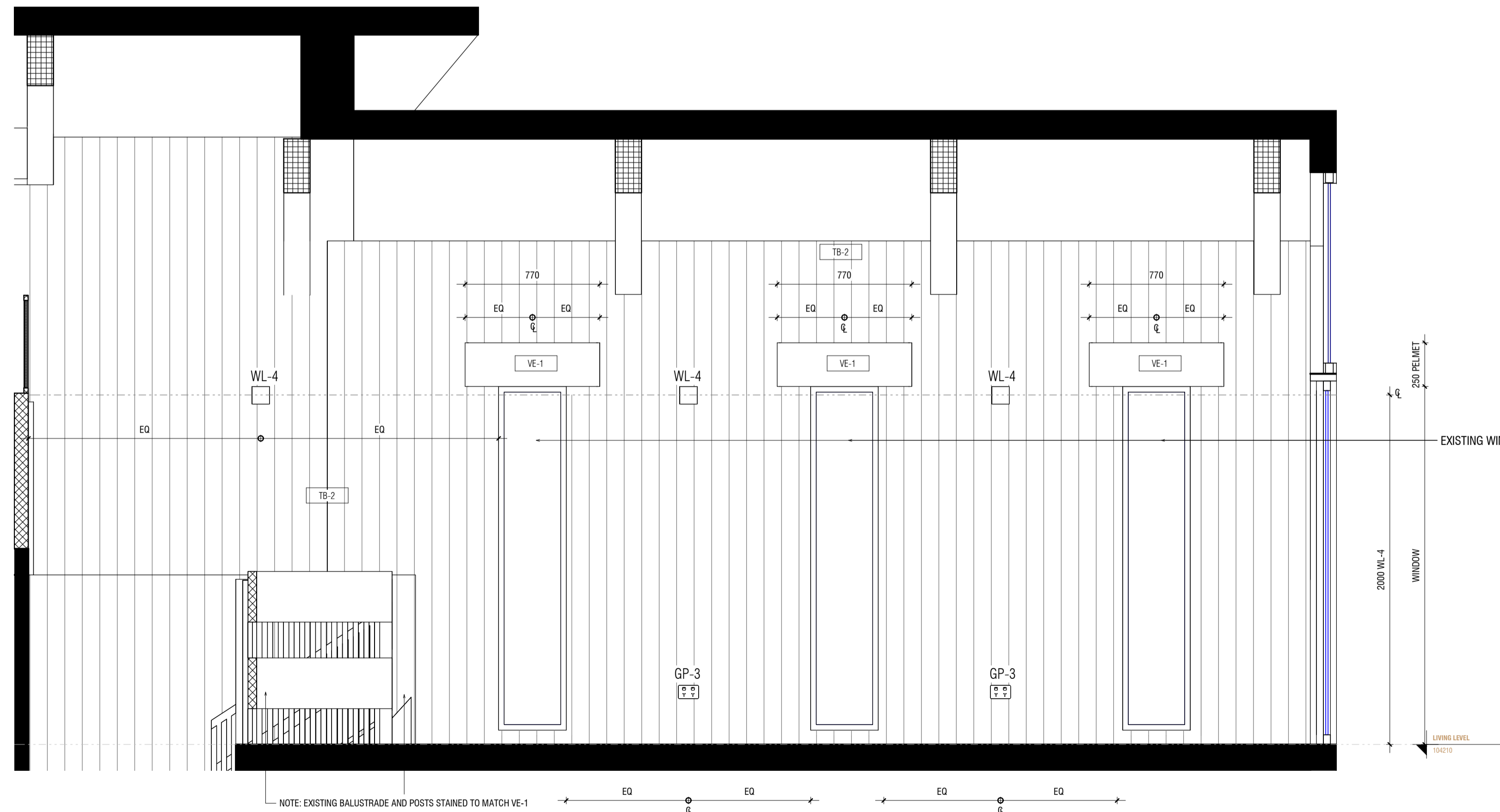
2 INT-5.02 ELEVATION 2 1 : 20
