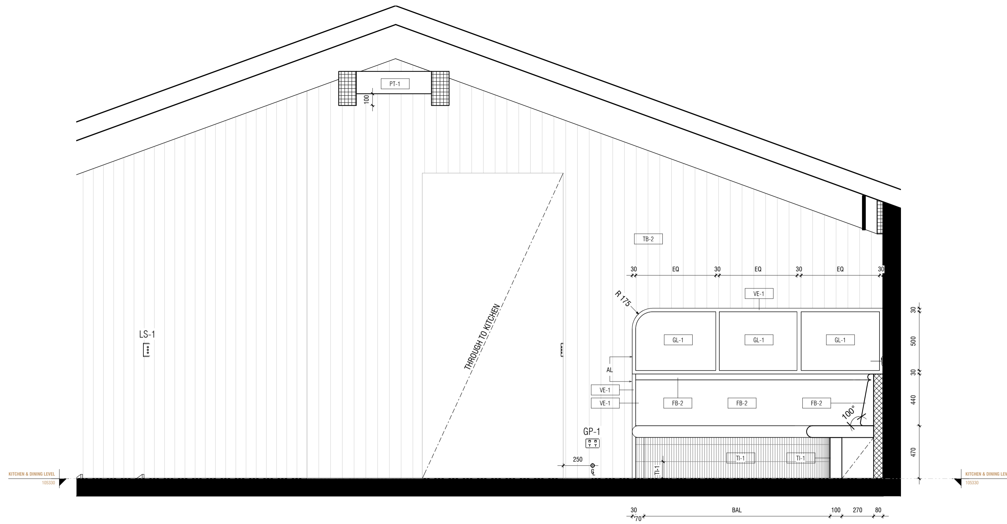
1 INT-4.02 ELEVATION 1 1:20
