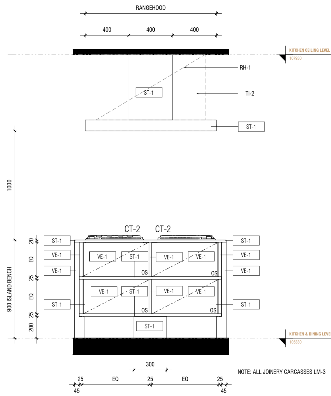
1 INT-3.05 ELEVATION 1 1 : 20
