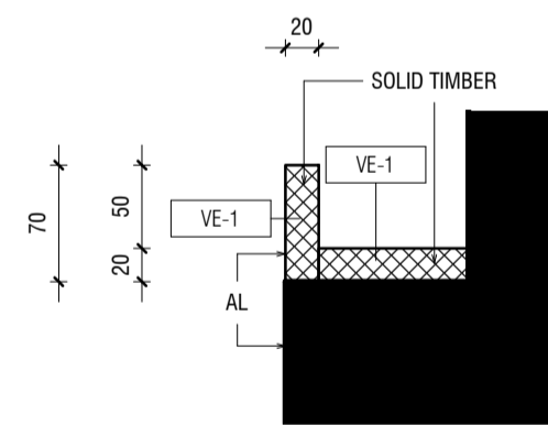
5 TOILET SHELF - SECTION 1:5
