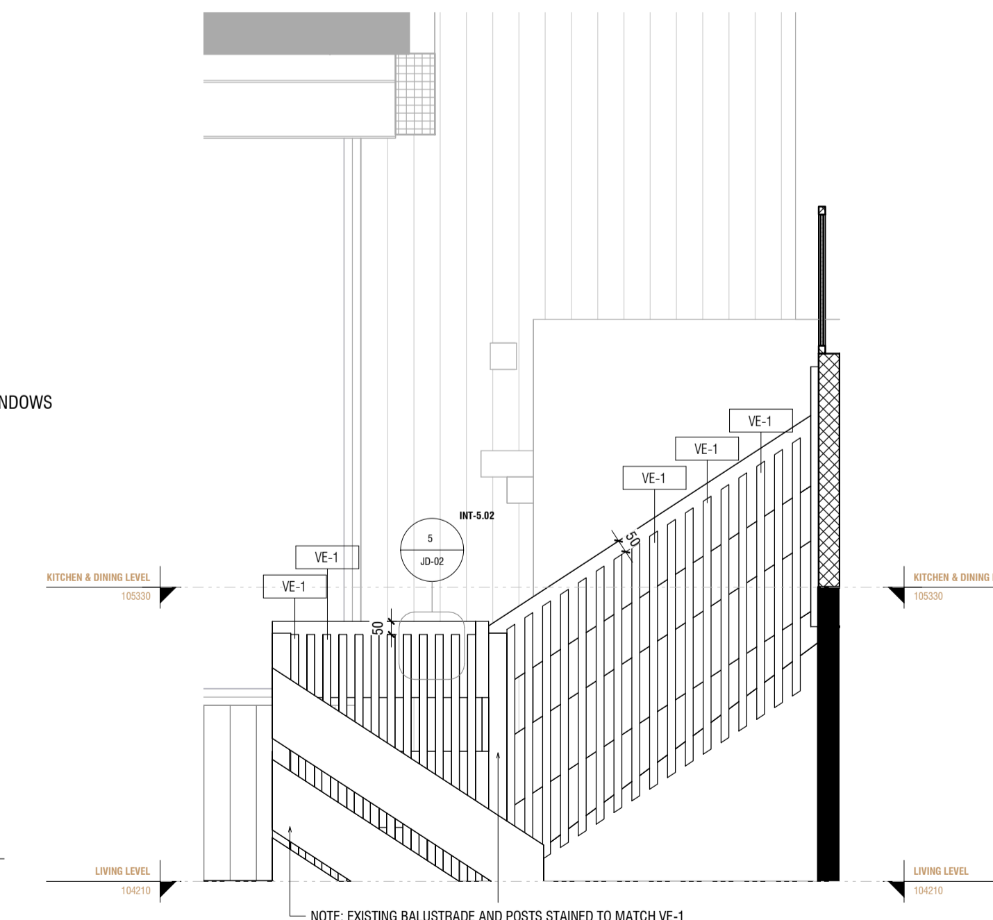
3 INT-5.02 ELEVATION 3 1 : 20
